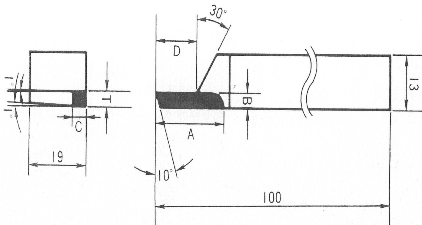
IE-30型形状图
