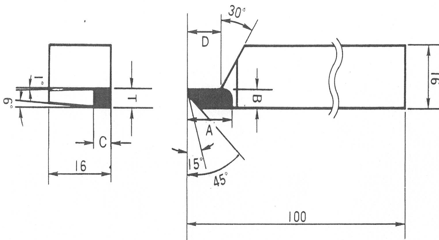
IE-20型形状图
